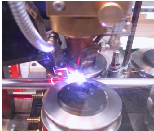
造管溶接
